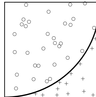
Rysunek 1: Ćwiartka koła w kwadracie.
